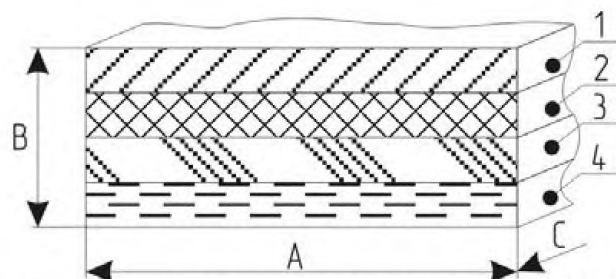
A – длина; B – толщина; C – ширина; 1 – специализированный абразивно-износостойкий слой; 2 – химостойкий слой; 3 – механически прочный слой; 4 – эластичный слой
