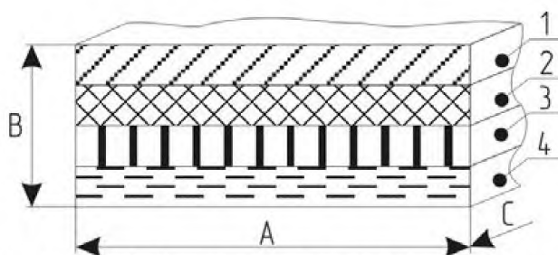
A – длина; B – толщина; C – ширина; 1 – специализированный химостойкий слой; 2 – химостойкий слой; 3 – механически прочный слой из металлической сетки, углеродной ткани или их аналогов (усиленный слой); 4 – эластичный слой
