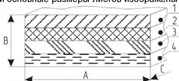
A – длина; B – толщина; C – ширина; 1 – специализированный химостойкий слой; 2 – химостойкий слой; 3 – механически прочный слой; 4 – эластичный слой
